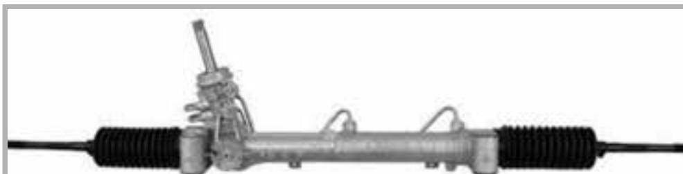
Lungh.1140 - Racc. filettati - Impianto TRW - Fabbr. TRW
