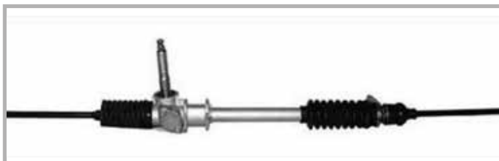
Lungh.1025 - Pign.110,5 - Tir. \varnothing 12x1,5 - att. ammort. alto
