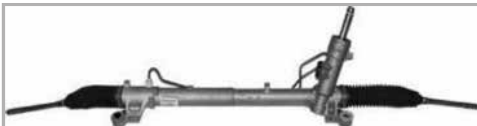
Lungh.1285 - Fabbr. TRW - Con cerchi 18
