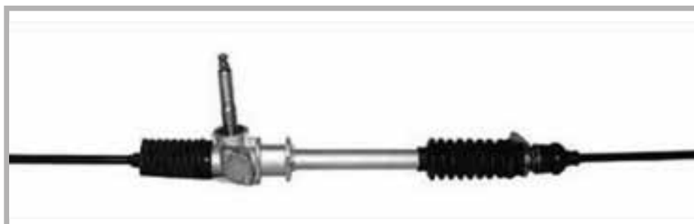
Lungh.1020 - Pign.110,5 - Tir. \varnothing 12x1,5
