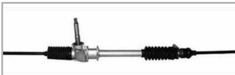
Lungh.1025 - Pign.110,5 - Tir. \varnothing 12x1,5 - att. ammort. basso
