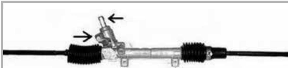
Lungh.1170 - Fabbr. Bendix - ZF - Foro ø10
