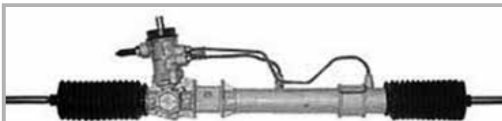
Lungh.1185 - Racc. ent.ø16/usc.ø16 - Tir. ø14x1,5 - Fabbr. SMI
